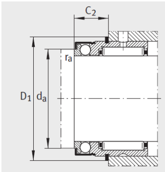
安装尺寸 外圈带卡环
