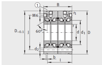
ZKLF...2RS-2AP ① 拉拔槽
