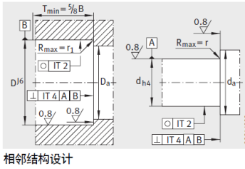
相邻结构设计
