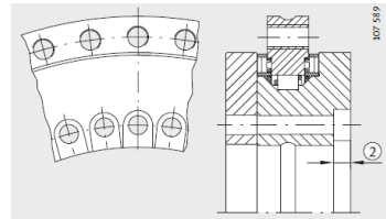
对于 YRTS325 ② 螺栓沉头孔开口方向 5)
