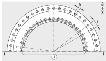
孔的分布 ① 两个保持螺栓
