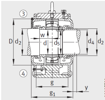
设计类型 B ③ 定位轴承 BF ④ 浮动轴承 BL
