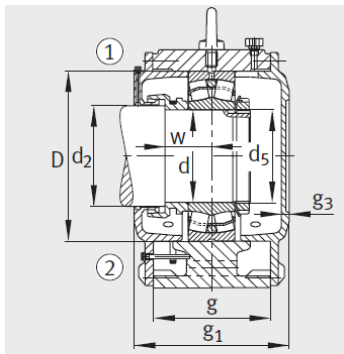
设计类型 A ① 定位轴承 AF ② 浮动轴承 AL
